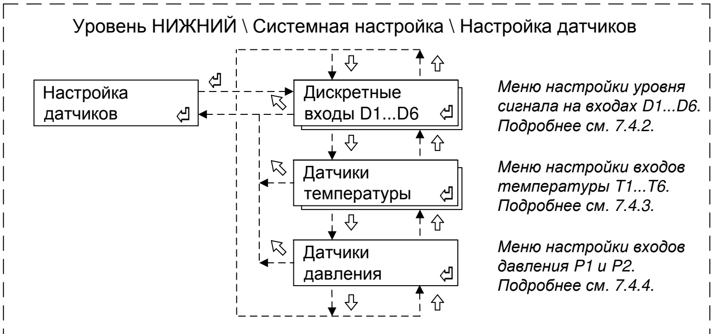
Рисунок 6 – Структура меню настройки датчиков (входов)
