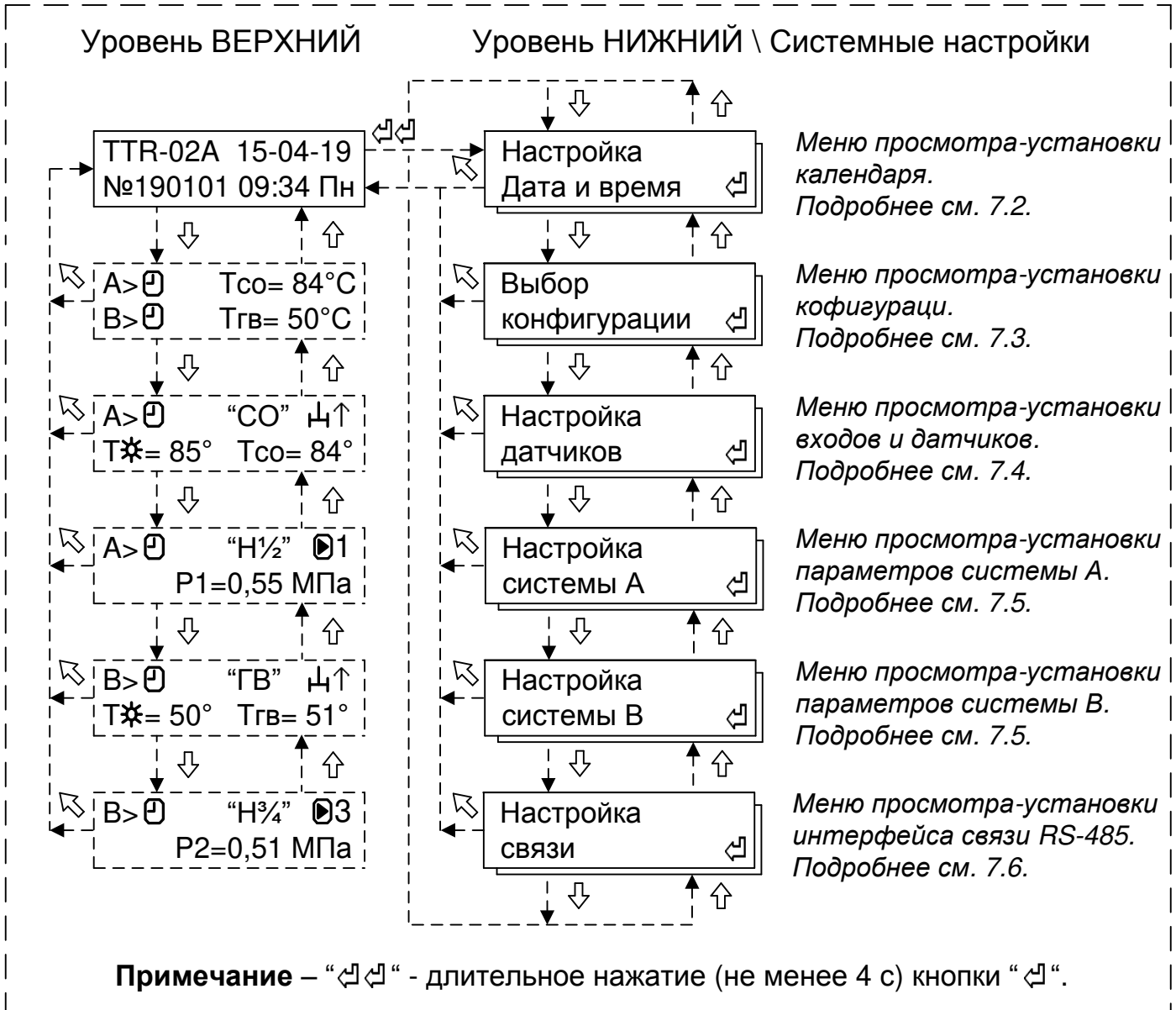
Рисунок 5 – Структура меню системной настройки
