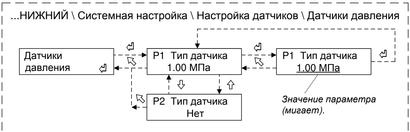
Рисунок 8 – Структура меню настройки датчиков давления
